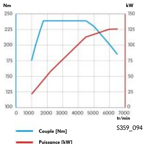
Moteur TSI de 1,4l/125kW
