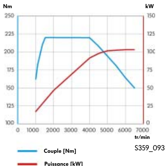
Moteur TSI de 1,4l/103kW
