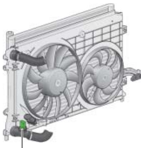
Transmetteur de température de liquide de refroidissement en sortie de radiateur G83
