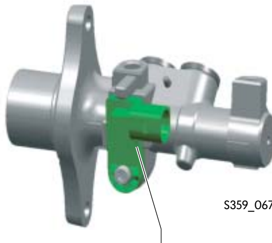
Transmetteur de position de pédale de frein G100
