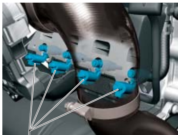
Injecteurs N30 - N33
